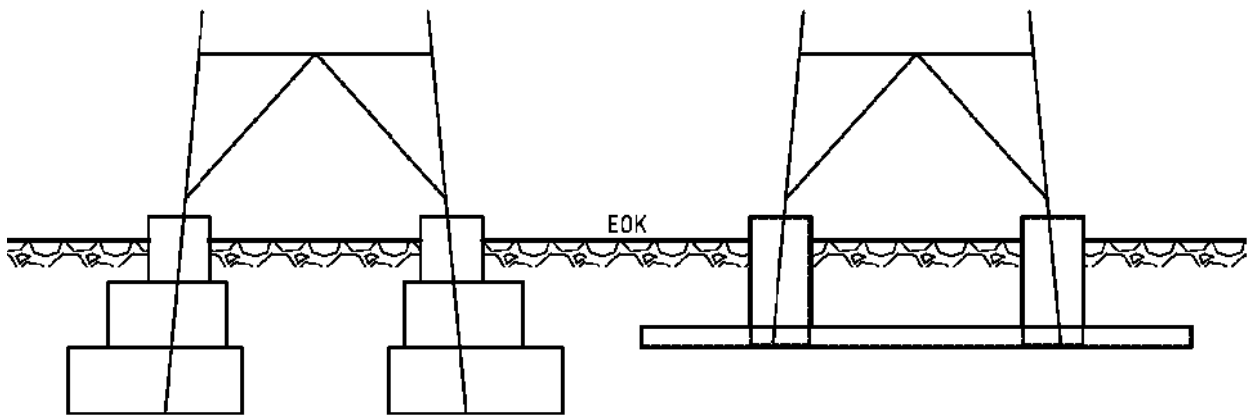
Stufenfundament
