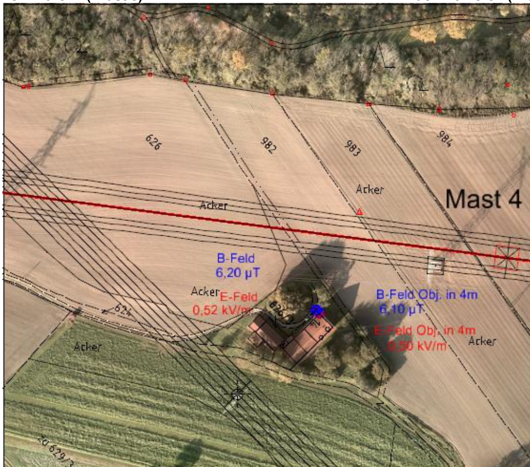
Maßstab 1:2000
