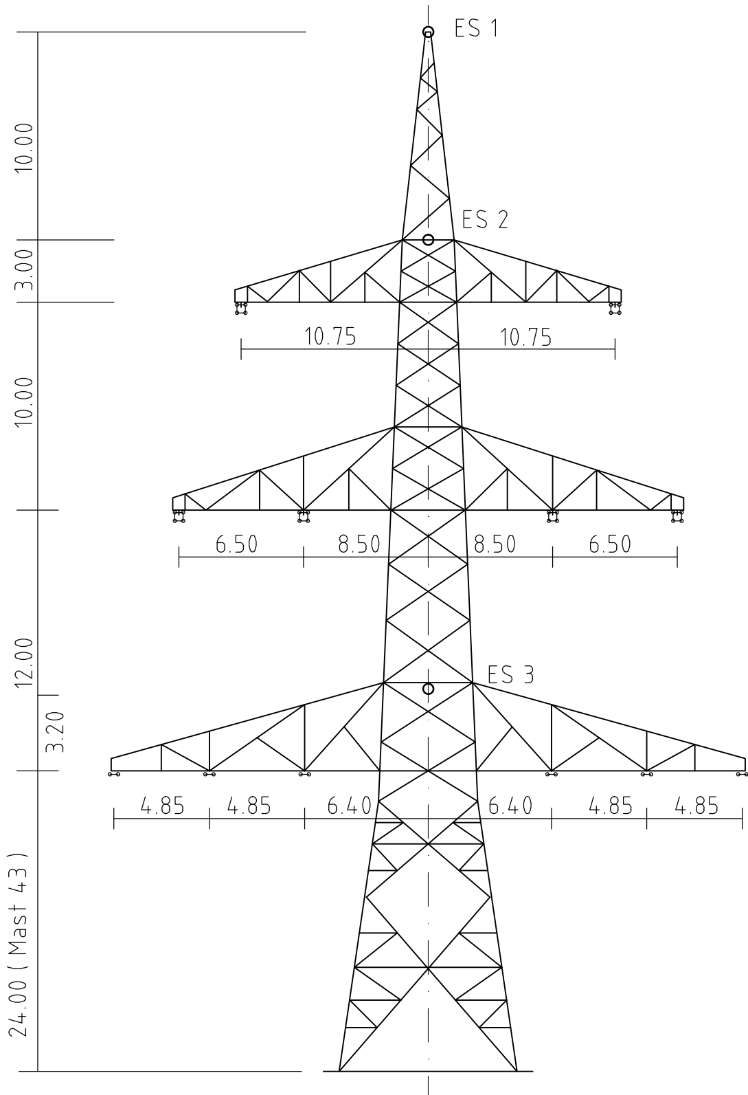
Mast Nr. 43
