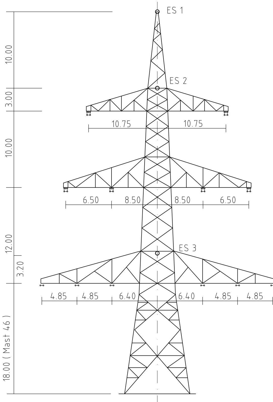
Mast Nr. 46
