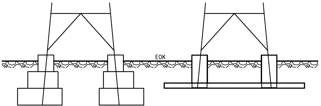
Stufenfundament
