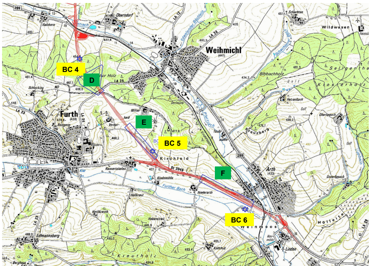
Abb. 1: Fledermaus-Untersuchung 2012: Lage der Probeflächen und Batcorder-Standorte
