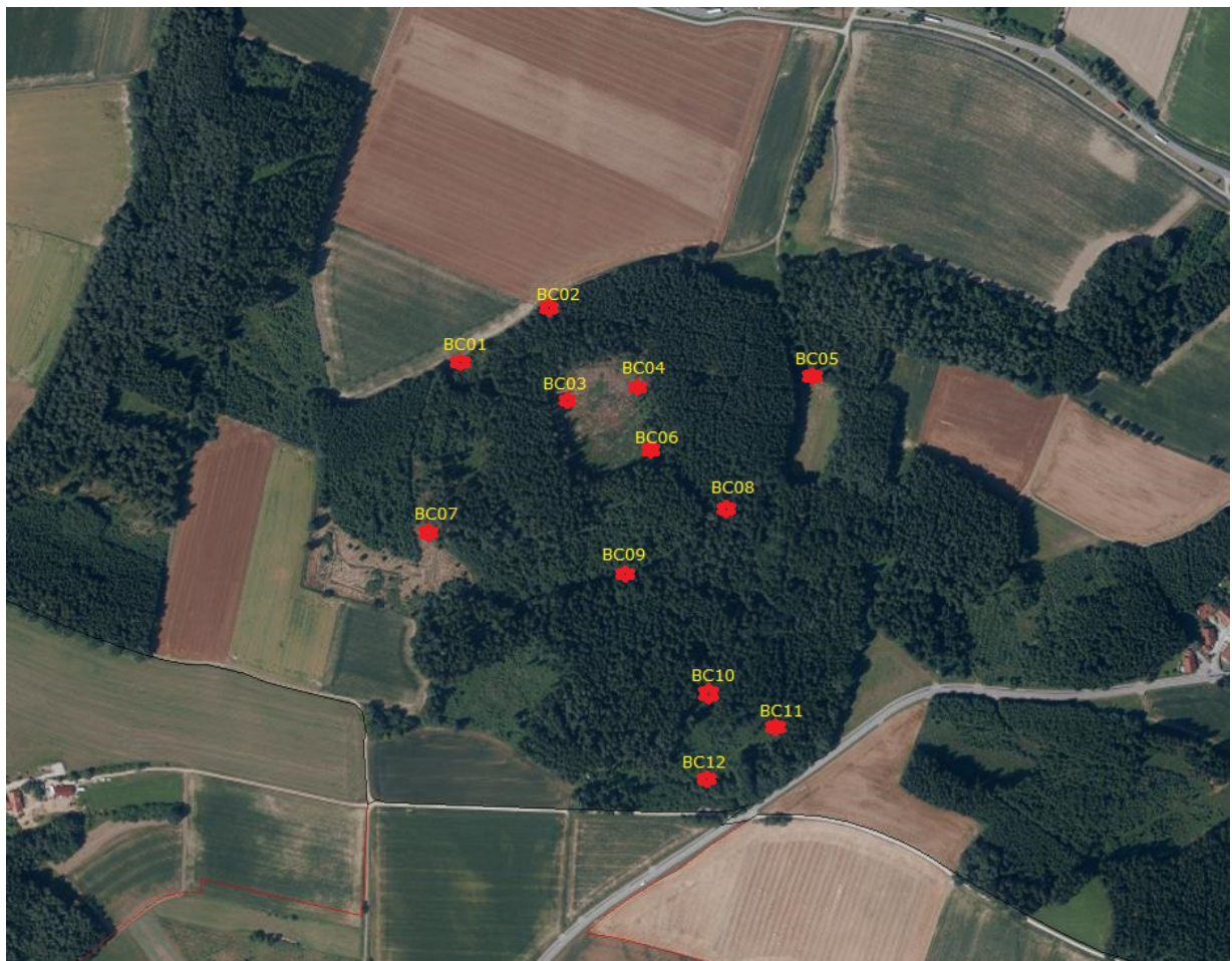
Abb. 2: Fledermaus-Untersuchung im Further Holz 2014: Lage der Batcorder-Standorte
