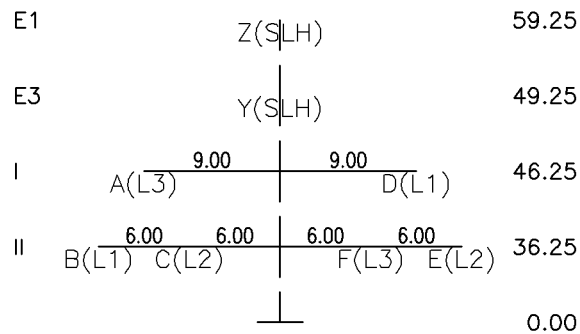
Mast Nr. 7
