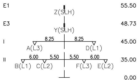
Mast Nr. 8
